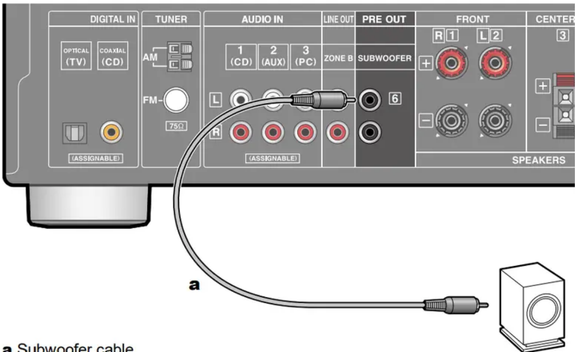
a Subwoofer cable
