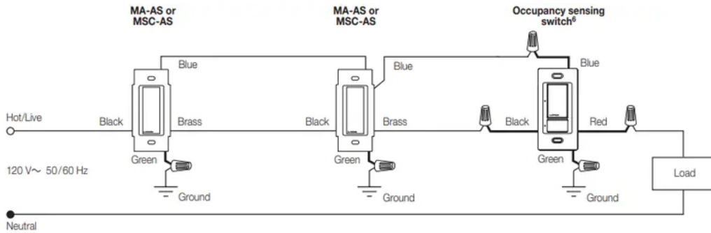
Wiring Diagram 15
