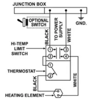
C-2 STANDARD SINGLE ELEMENT 120 VOLT & 277 VOLT
