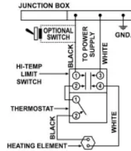
C-2 STANDARD SINGLE ELEMENT 120 VOLT & 277 VOLT
