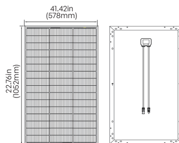
RSP120DC-ASR
