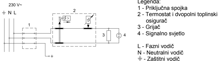
Električna spojna shema
