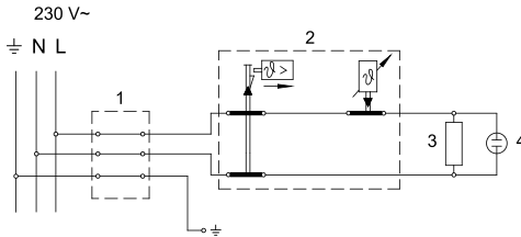
Elektroschaltbild
