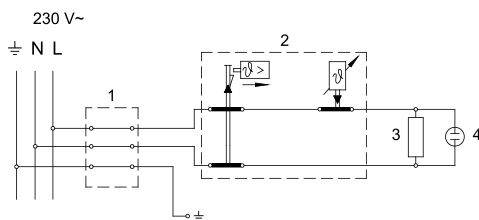
Шема на електрично поврзување
