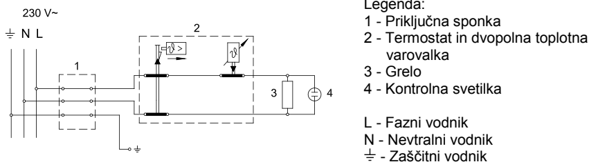
Shema električne vezave
