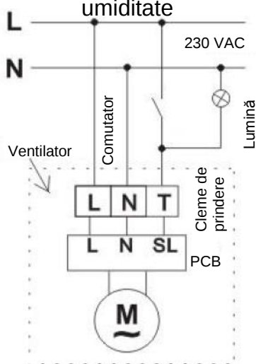
Schemă pentru cablare - modele cu temporizator/senzor de umiditate
