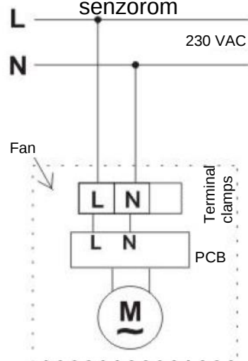
Schéma zapojenia s pohybovým senzorom
