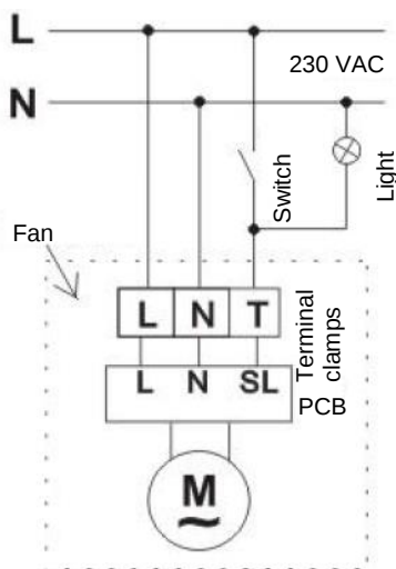
zapojenie – modely s časovačom/senzorom vlhkosti
