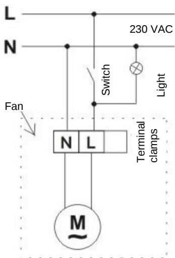
Schéma zapojenia – štandardné modely
