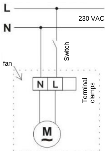
Schéma zapojenia – štandardné modely
