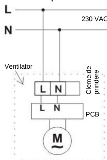
Schemă pentru cablare cu senzor de mișcare
