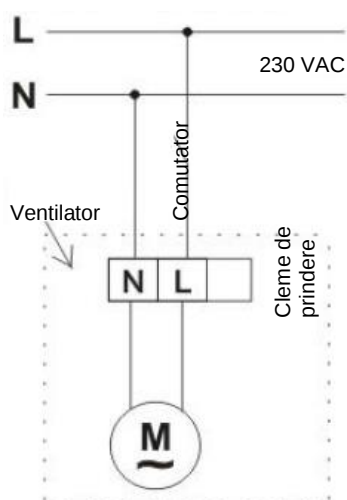
Schemă pentru cablare - modele standard
