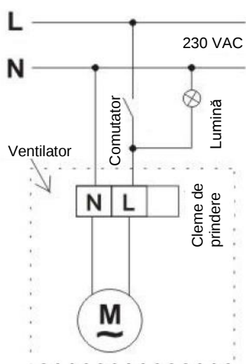
Schemă pentru cablare - modele standard
