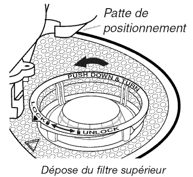
Dépose du filtre supérieur
