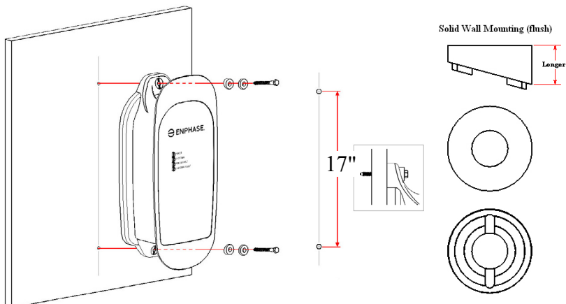
Figura 9: Montaje del EVSE en una pared sólida
