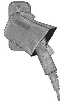
Figure 13 : Cadenas utilisé en combinaison avec l'étui du connecteur après la charge
