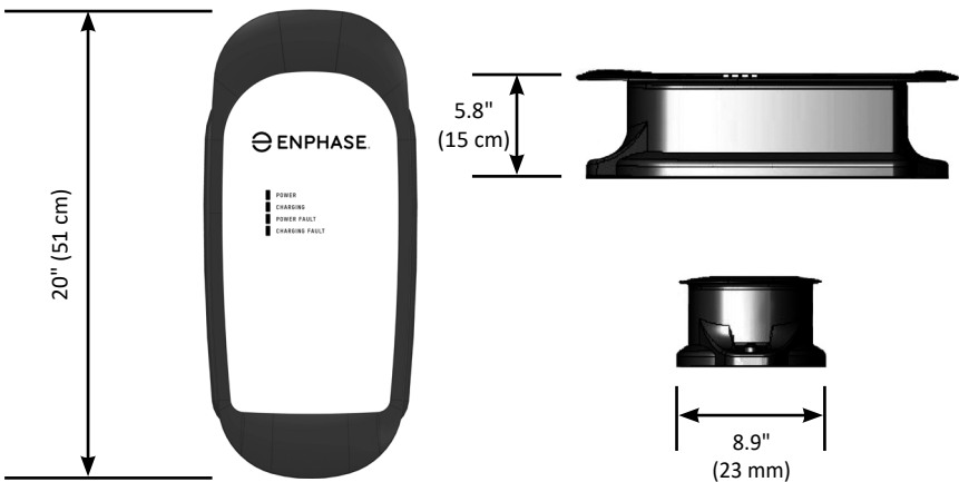
Figure 14 : Dimensions du boîtier
