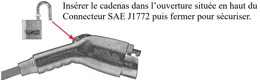
Figure 11 : Verrouillage du connecteur SAE J1772 avec cadenas inclus
