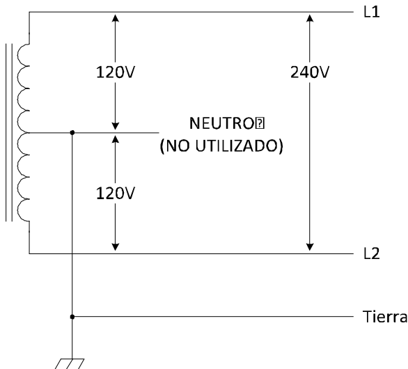
Figura 3: Monofásico de 220/240V
