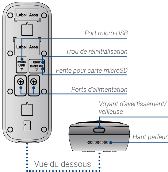
Panneau arrière
