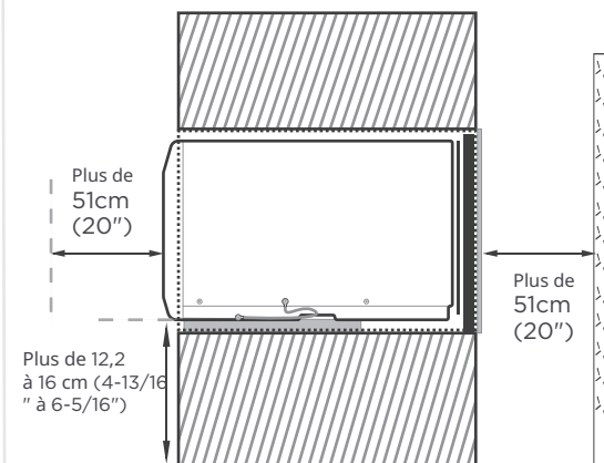
Vue latérale
