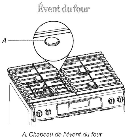
A. Chapeau de l'évent du four
