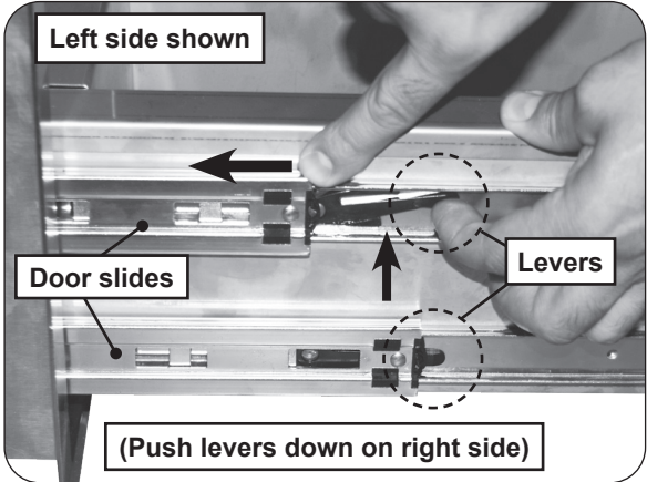
Fig. 1-2 Door removal
