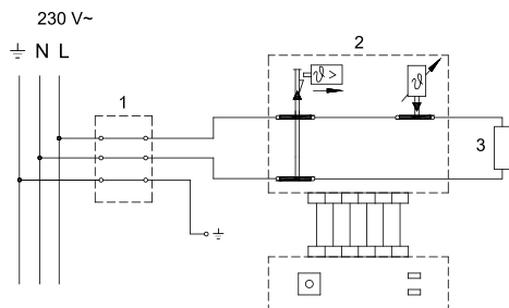
Električna spojna shema
