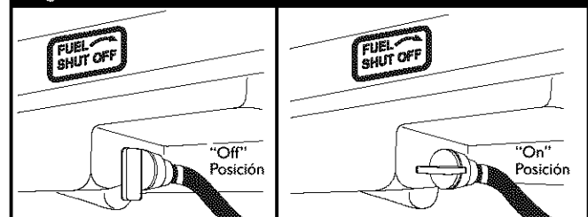
Figura 10 — Válvula de Combustible
