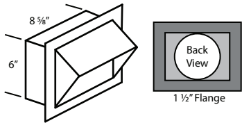
WALL LOUVER
