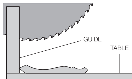
MOULURE COURONNÉE À PLAT SUR LA TABLE CONTRE LE GUIDE
