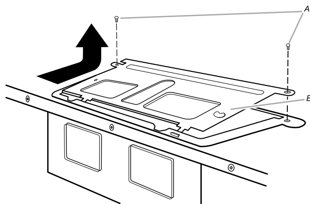
A. Screws B. Damper plate
