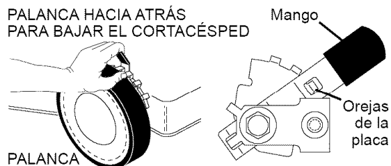
PALANCA HACIA ATRÁS PARA BAJAR EL CORTACÉSPED PALANCA HACIA ADELANTE PARA LEVANTAR EL CORTACÉSPED
