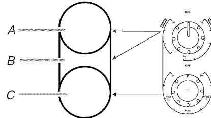
A. Dimension simple B. Zone de pont C. Dimension simple
