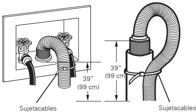
Sujetacables
