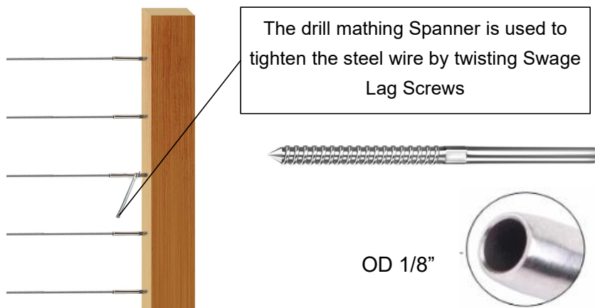
Accesorio para poste de madera
