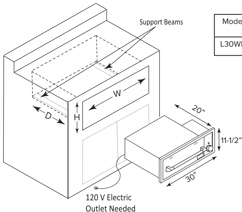
Cutout Dimensions
