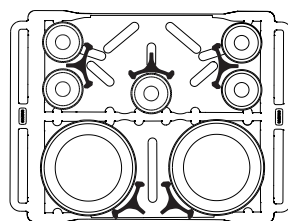
2 стопы: диам. от 23,5 см до 33 см (по 45–60 шт.) 5 стоп: диам. 12,6 см (по 45–60 шт.) Общая вместимость: 345–390 шт.
