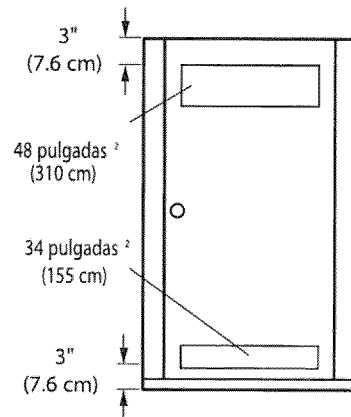
Requisitos de ventilación de la puerta del armario
