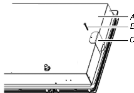
A. Partie inférieure de la base de la table de cuisson B. Vis de fixation C. Bride de fixation (emplacements d'extrémité recommandés)
