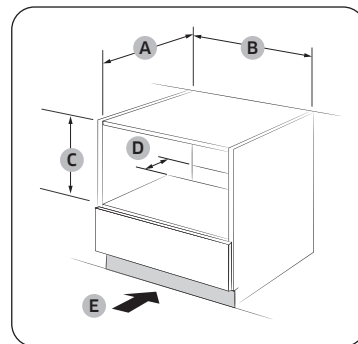
Unterbauschränk (mm)
