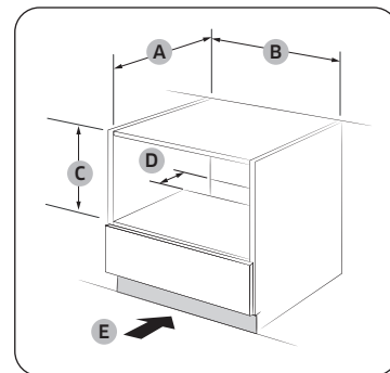
Allaskaappi (mm)
