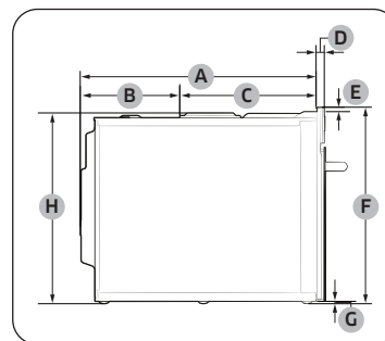
Ugn (mm)
