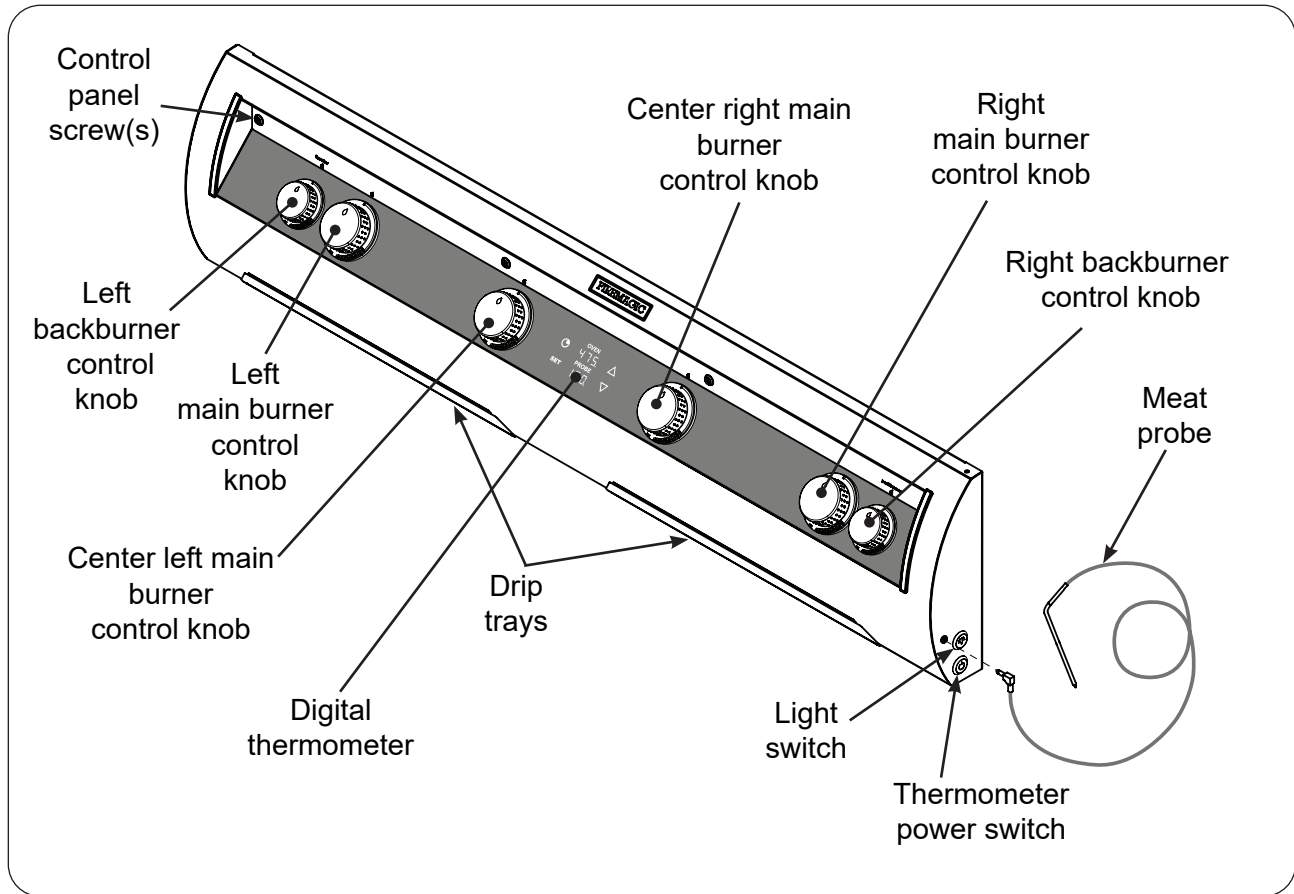
Fig. 34-1 E1060i controls
