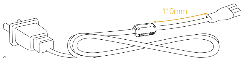
圖1 安裝磁環
