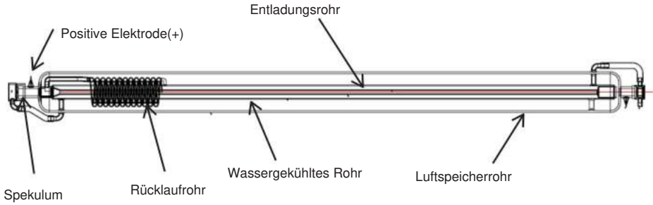
Laser-Outlet
