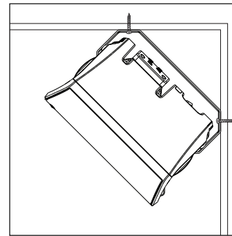
FIGURA 15: Instalación del soporte a 45°.
