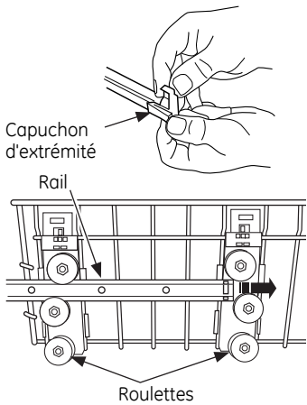
Panier supérieur - 8 couverts - GDF510, GDF520 & ADT521
