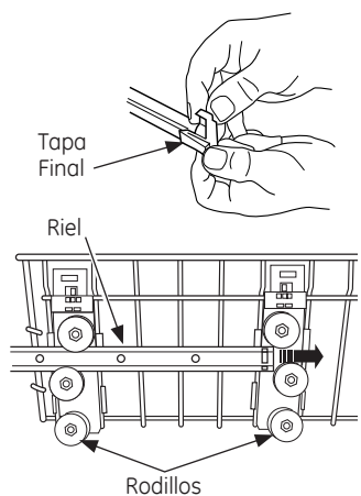
Estante Superior-Configuraciones de 8 lugares - GDF510, GDF520 & ADT521
