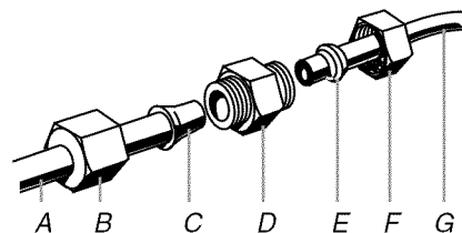
A. Conduit vers le réfrigérateur B. Écrou (fourni) C. Rénflement D. Raccord (à acheter) E. Virole (à acheter) F. Écrou (à acheter) G. Canalisation d'eau du domicile
