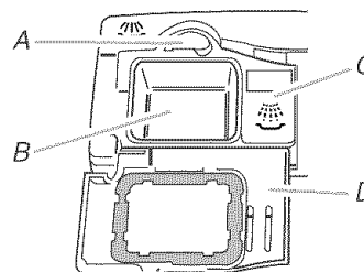
A. Loquet du couvercle B. Section du lavage principal C. Section du prélavage D. Couvercle
