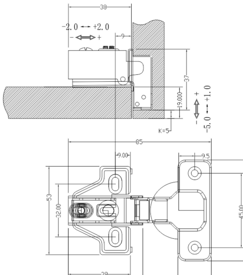
ÿ35 CLIP ON EENWEG HYDRAULISCHE BUFFERING SCHARNIEREN
