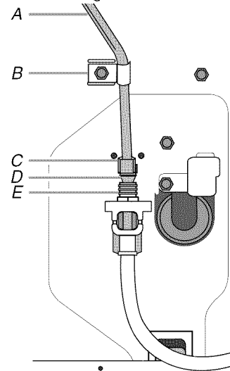
A. Tube en cuivre B. Bride en "P" C. Écrou de compression D. Bague de compression E. Valve d'entrée d'eau
