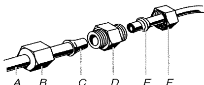
A. Tubería de agua al refrigerador B. Tuerca (provista) C. Bulbo D. Acoplamiento (provisto) E. Férula (adquirida) F. Tuerca (adquirida)
