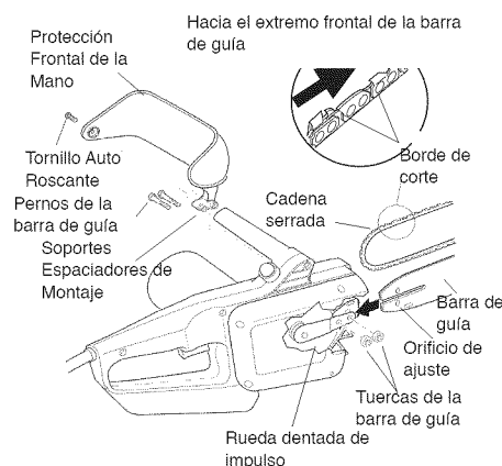
Figura 2 - Ensamble de la Barra Guía, Cadena y Protección para la mano
