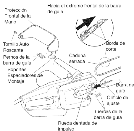
Figura 4 - Ensamble de la Barra Guía, Cadena y Protección para la mano
