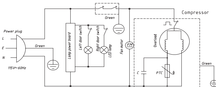
Diagrama de cableado
