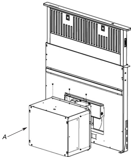
A. Caisse du moteur de ventilateur
