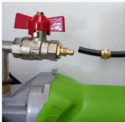
3. Instale las juntas de las tuberías de agua y fíjelas con una llave.
