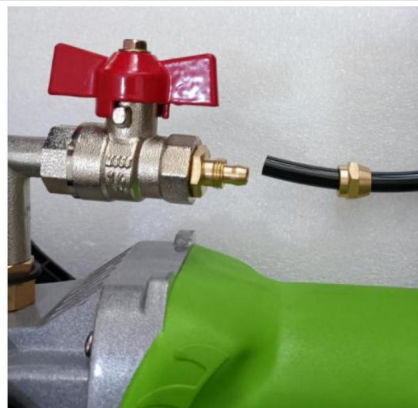
3. Installare i giunti del tubo dell'acqua, bloccarli con una chiave.
