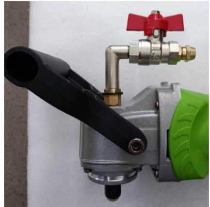
2. Installeer de waterklep
