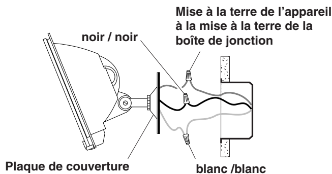
Câblage du Luminaire (Le produit pourrait être différent de l'illustration)
