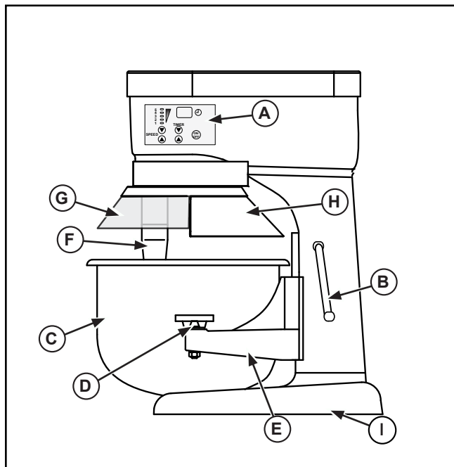
Abbildung 1. 6,6- und 11-l-Mixer – Funktionsmerkmale und Bedienelemente.
