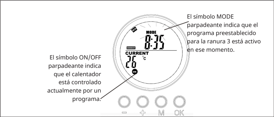
Visualización en la página del sistema cuando el programa está en marcha
