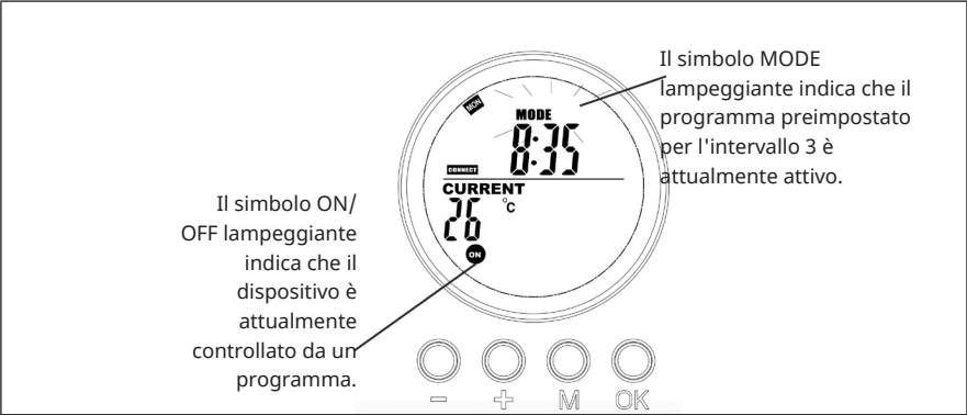
Visualizzazione nella pagina di sistema quando il programma è in esecuzione
