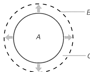
A. Zone de cuisson à la surface B. Ustensile de cuisson/autoclave C. Dépassement maximal 1" (2,5 cm)
