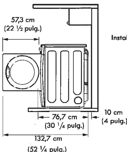
Instalación estándar – Vista lateral
