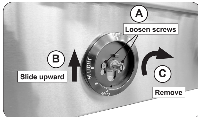
Fig. 40-2 Remove bezels
