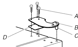
A. Vis de charnière à tête hexagonale de \frac{5}{16} " B. Charnière supérieure C. Axe de charnière D. Cale
