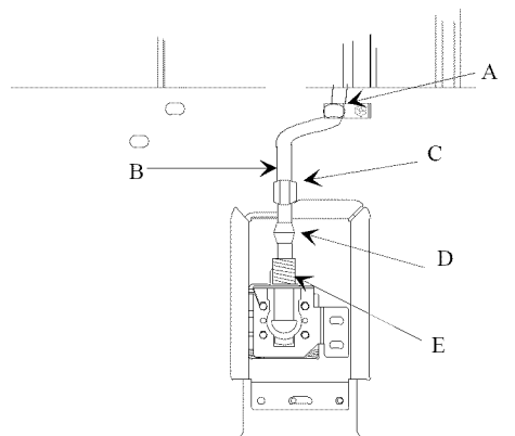
Raccord de conduite d'eau
