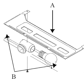
B. Ampoule électrique
