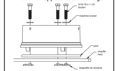
Vue latérale de la buse monter sur le haut de l'appareil de chauffage
